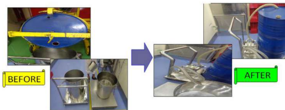
Gambar 5. Perbandingan Sebelum dan Setelah Penggunaan Rancangan Alat Bantu Sumber : Pengolahan data, 2020
