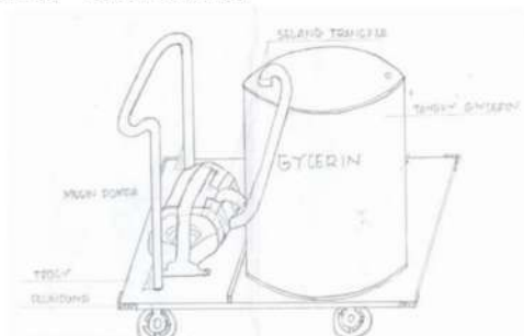
Gambar 3. Rancangan Alat Bantu Penimbangan Glycerin Sumber : Pengolahan data, 2020
