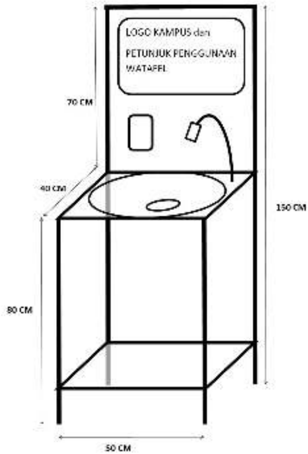
Gambar 3. 1 Rancangan Wastafel
