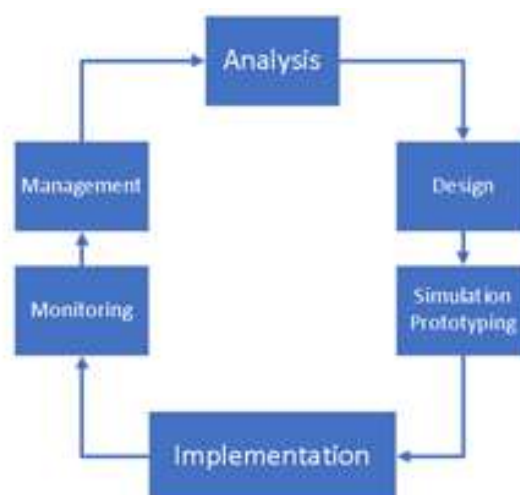
Gambar 1. Tahapan NDLC
