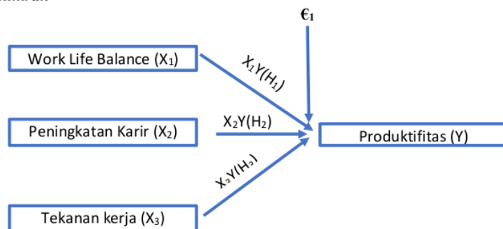
Gambar 1. Kerangka Riset Sumber: Data Primer, SmartPLS 3.0, 2021
