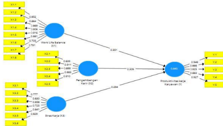
Gambar 2. Diagram Jalur Riset Sumber: Data Primer, SmartPLS 3, 2021
