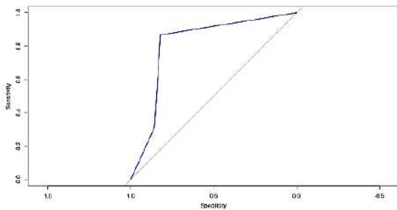
Gambar 3. Kurva ROC Klasifikasi Naive bayes
