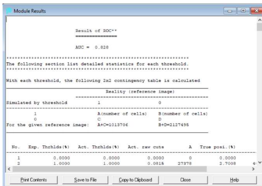
Gambar 5. Hasil Validasi
