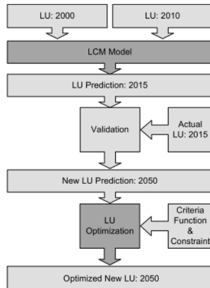
Gambar 3. Proses Prediksi
