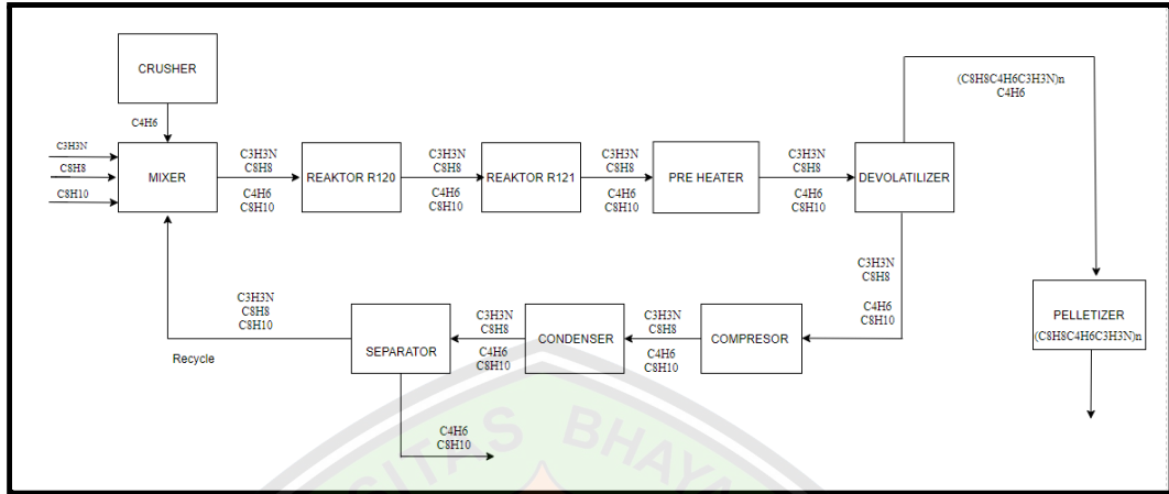
Gambar 1.9. Diagram Alir Kualitatif Proses Produksi ABS
