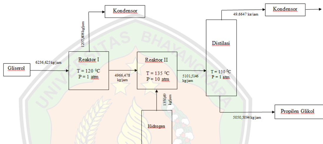
Gambar 1.7. Diagram Alir Kuantitatif Pabrik Propilen Glikol
