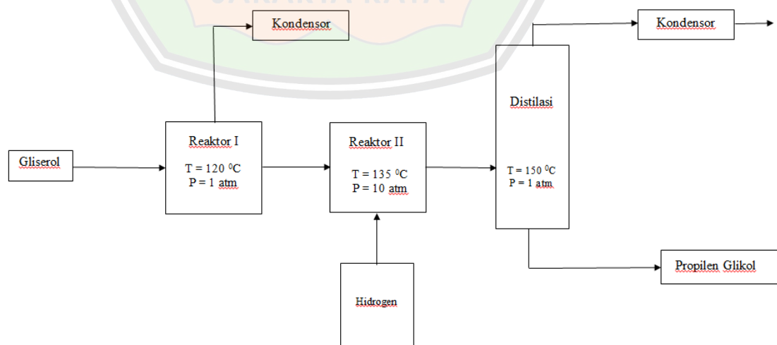
Gambar 1.6. Diagram Alir Kualitatif Pabrik Propilen Glikol
