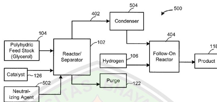
Gambar 1.5. Produksi propilen glikol pada Paten US 7943805 B2
