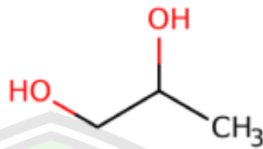
Gambar 1.2. Struktur Propilen Glikol
