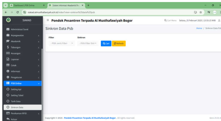
Gambar 3. Integrasi Data
