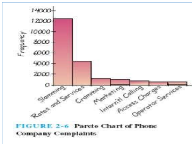
Gambar 2.4 Grafik pareto
