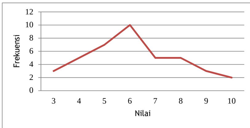
Gambar 2.1 Grafik Poligon frekuensi
