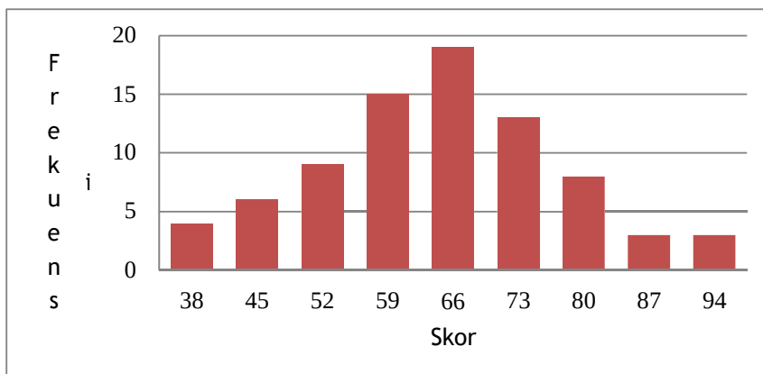
Gambar 2.2 Grafik Histogram
