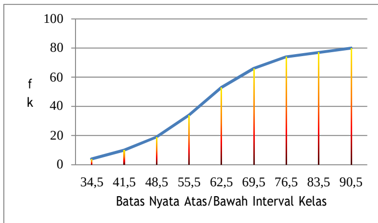
Gambar 2.3 Grafik ogif untuk contoh data pada tabel 3.5
