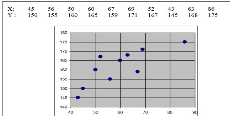
Gambar 2.6 Grafik pencar
