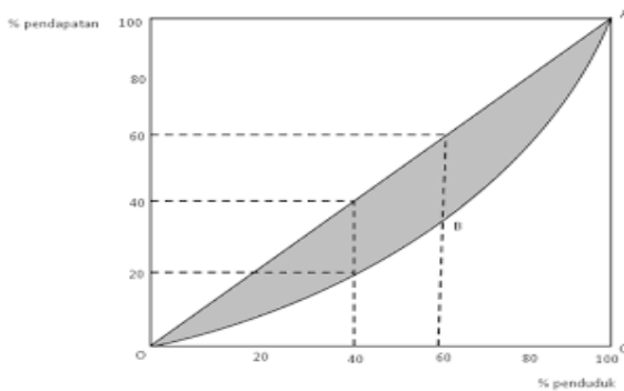
Gambar 1. Kurva Lorenz
