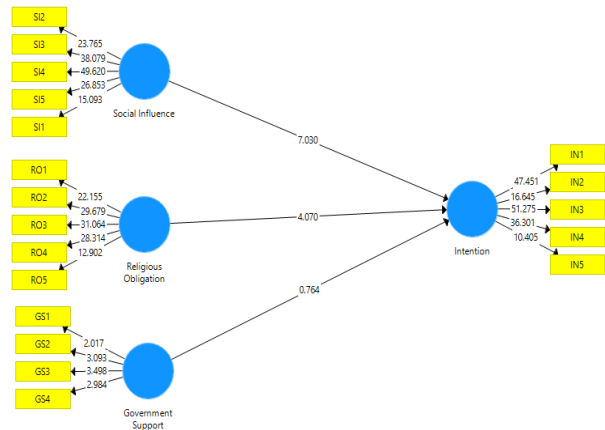
Gambar 3 Uji Hipotesis
