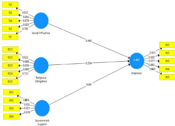
Gambar 2 Validitas Data
